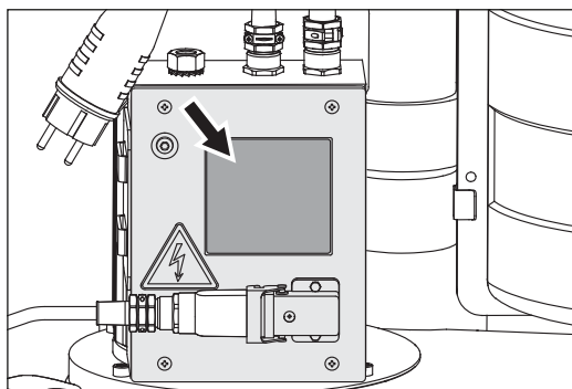
Fig. 1 Placa de identificación en la tapa de la caja de distribución del motor.
