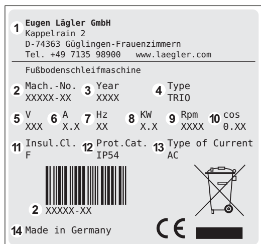
Fig. 2 Datos en placa de identificación (véase el texto principal).
