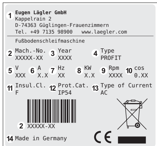
Fig. 3 Datos en placa de identificación (véase el texto principal).
